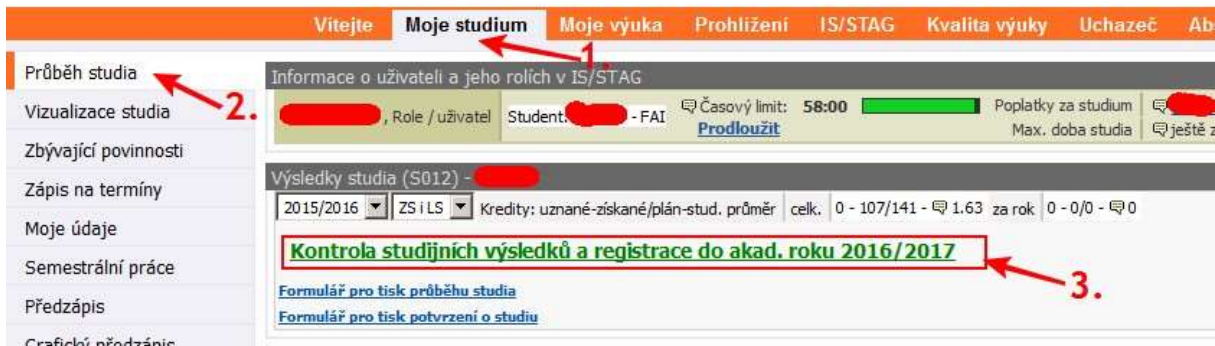
Obr. 1 Portál IS/STAG
